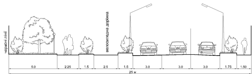
ПРОФІЛЬ VII-VII
