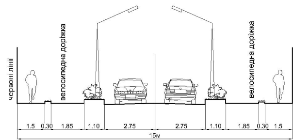
ПРОФІЛЬ II-II
