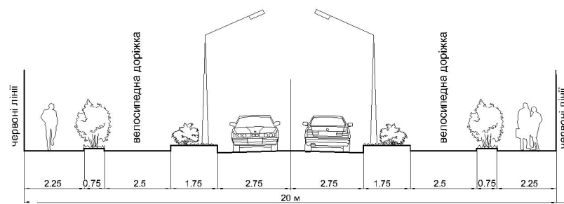
ПРОФІЛЬ IV-IV
