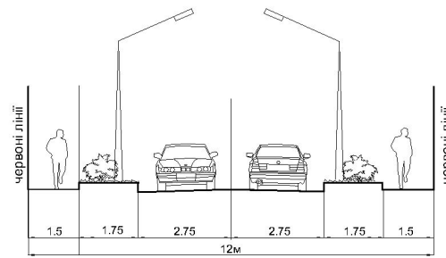
ПРОФІЛЬ I-I
