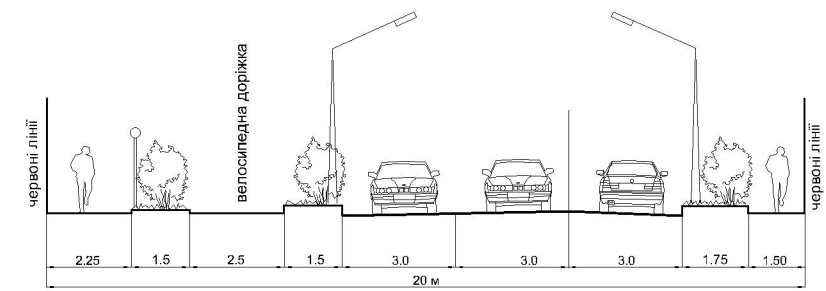
ПРОФІЛЬ VI-VI
