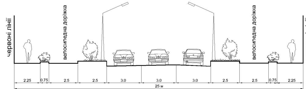
ПРОФІЛЬ VIII-VIII
