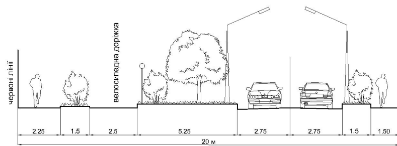
ПРОФІЛЬ V-V
