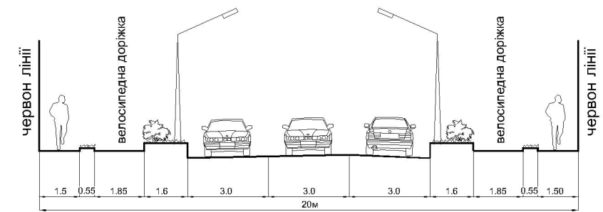
ПРОФІЛЬ III-III
