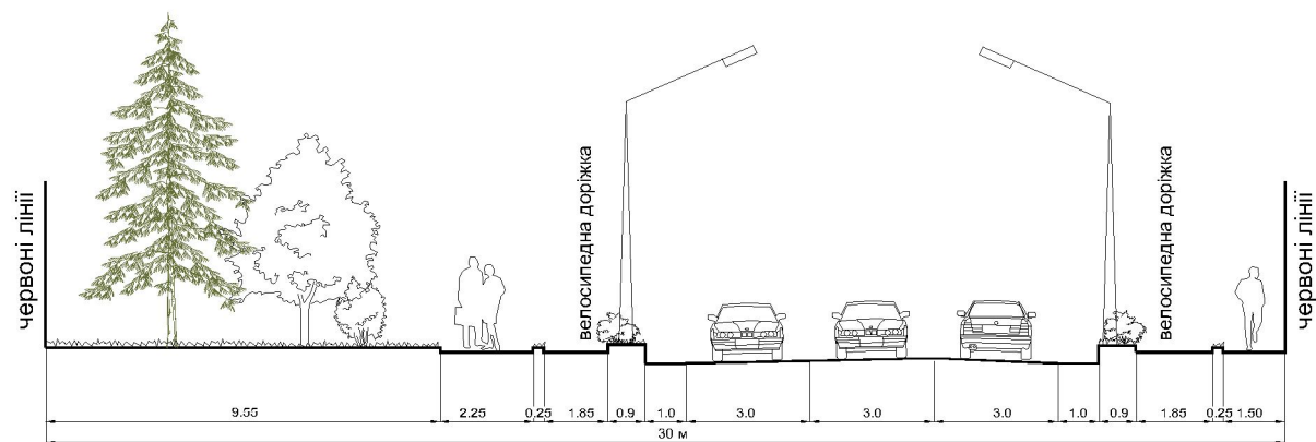
ПРОФІЛЬ IX-IX
