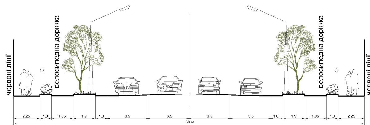
ПРОФІЛЬ X-X
