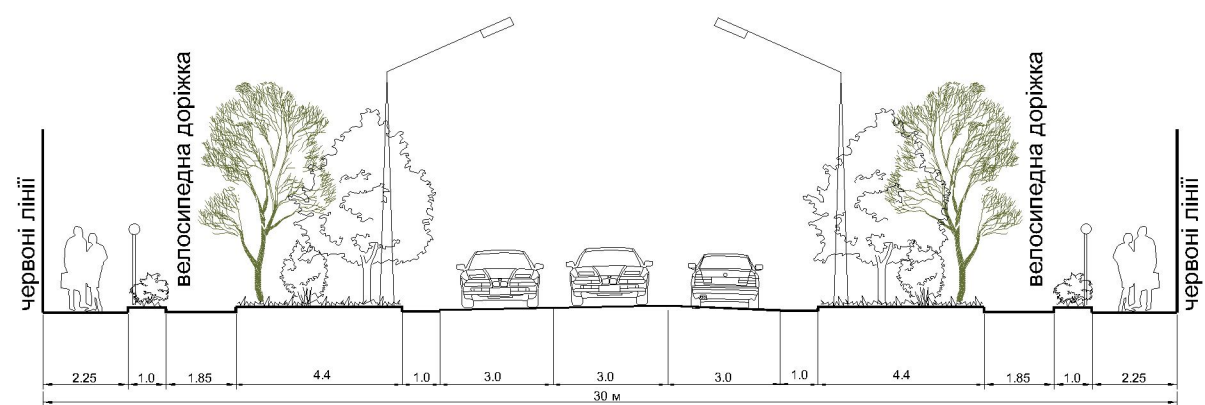
ПРОФІЛЬ XI-XI
