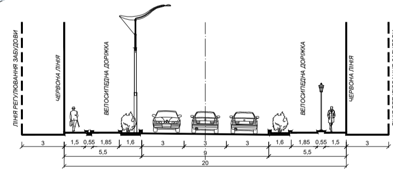
ПРОФІЛЬ II-II (вул. Молодіжна)
