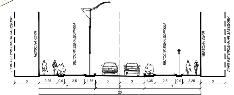
ПРОФІЛЬ III-III (вул. М. Гоголя)
