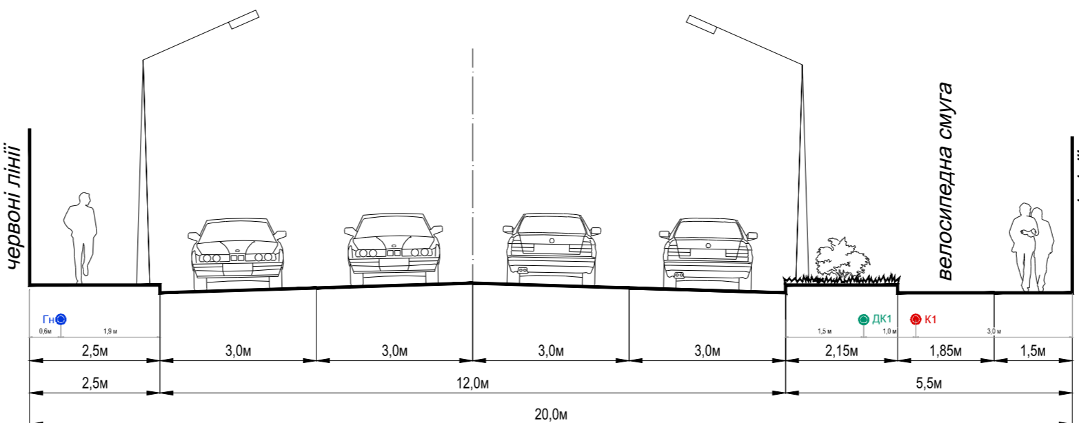
ПРОФІЛЬ ІІ-ІІ
