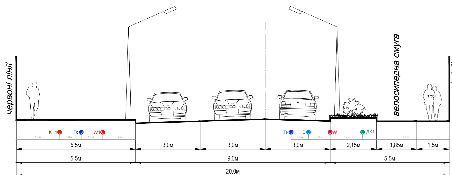
ПРОФІЛЬ І-І
