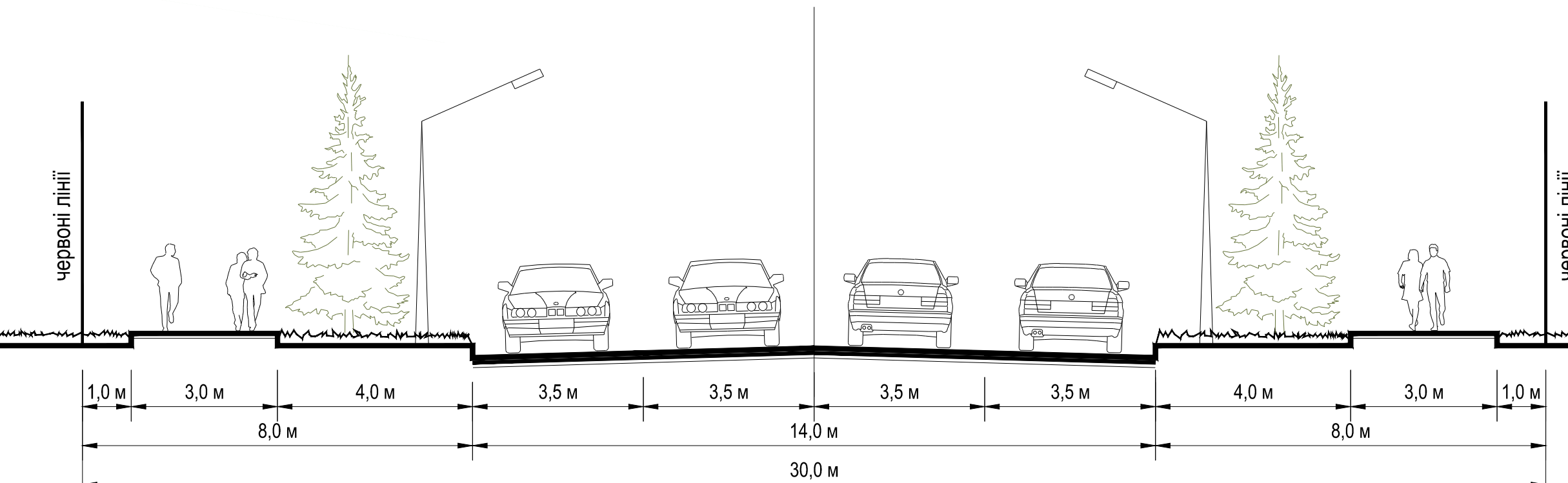
ПОПЕРЕЧНІ ПРОФІЛІ ВУЛИЦЬ М 1:100
