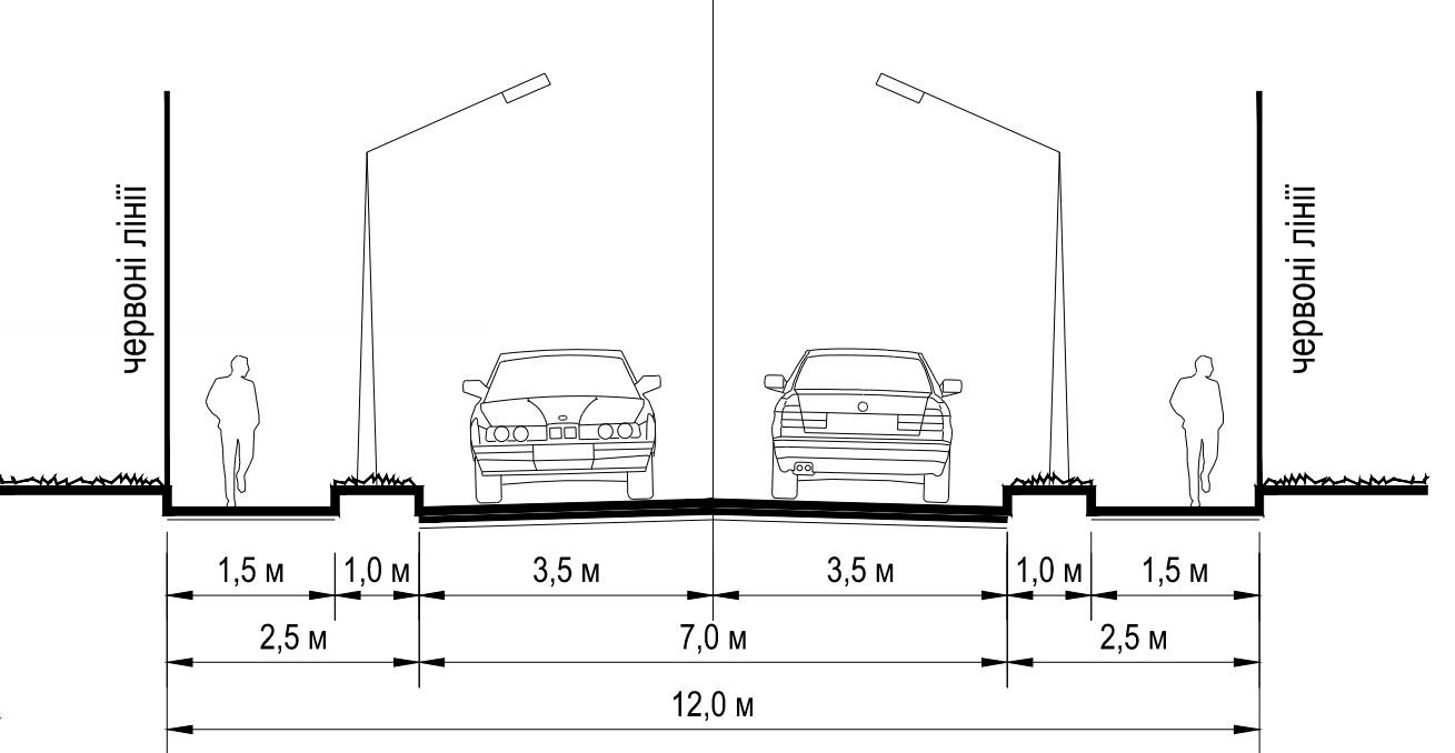
ПРОФІЛЬ III-III
