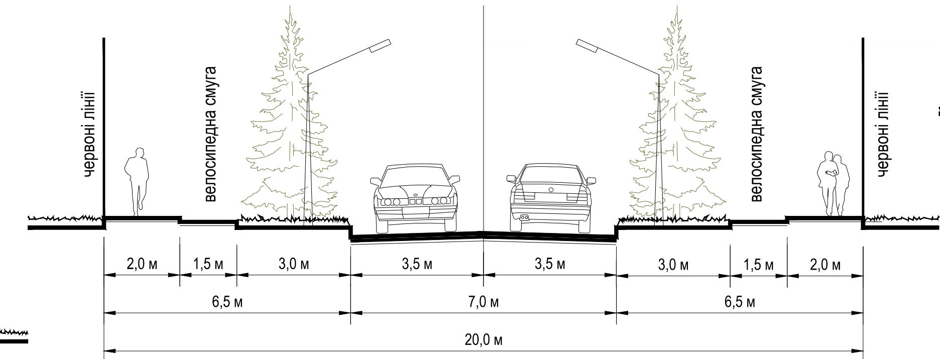
ПРОФІЛЬ II-II
