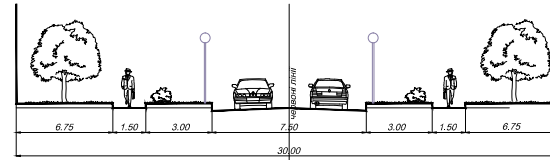
ПРОФІЛЬ І-І:
