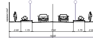
ПРОФІЛЬ ІІ-ІІ:
