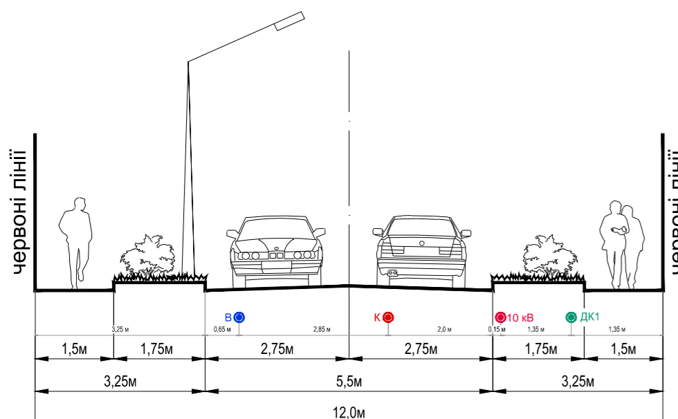
ПРОФІЛЬ І-І
