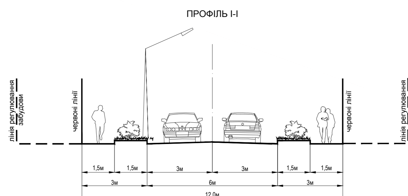
ПРОФІЛЬ І-І
