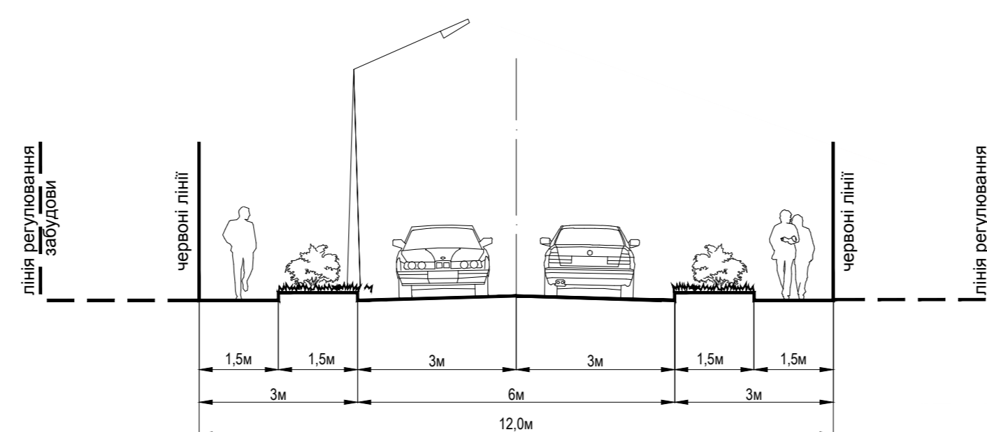
ПРОФІЛЬ І-І
