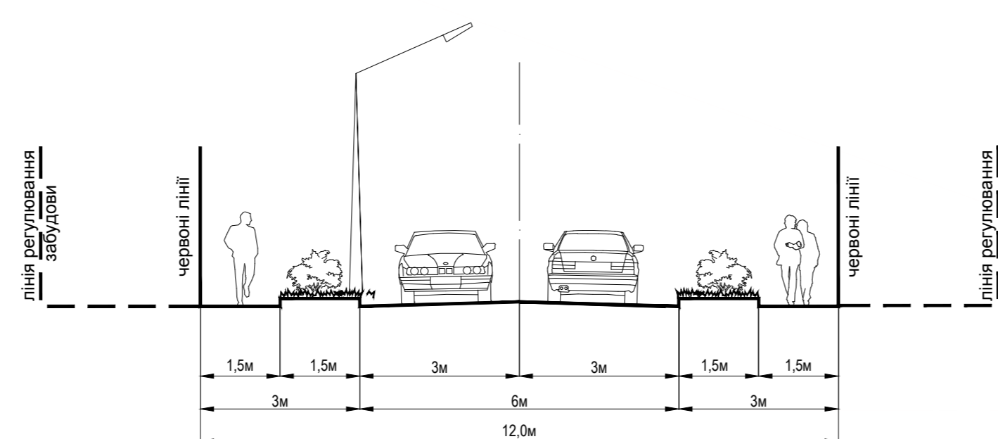
ПРОФІЛЬ І-І
