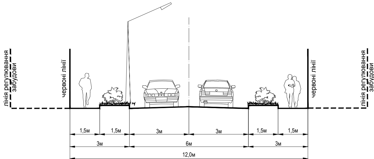
ПРОФІЛЬ І-І
